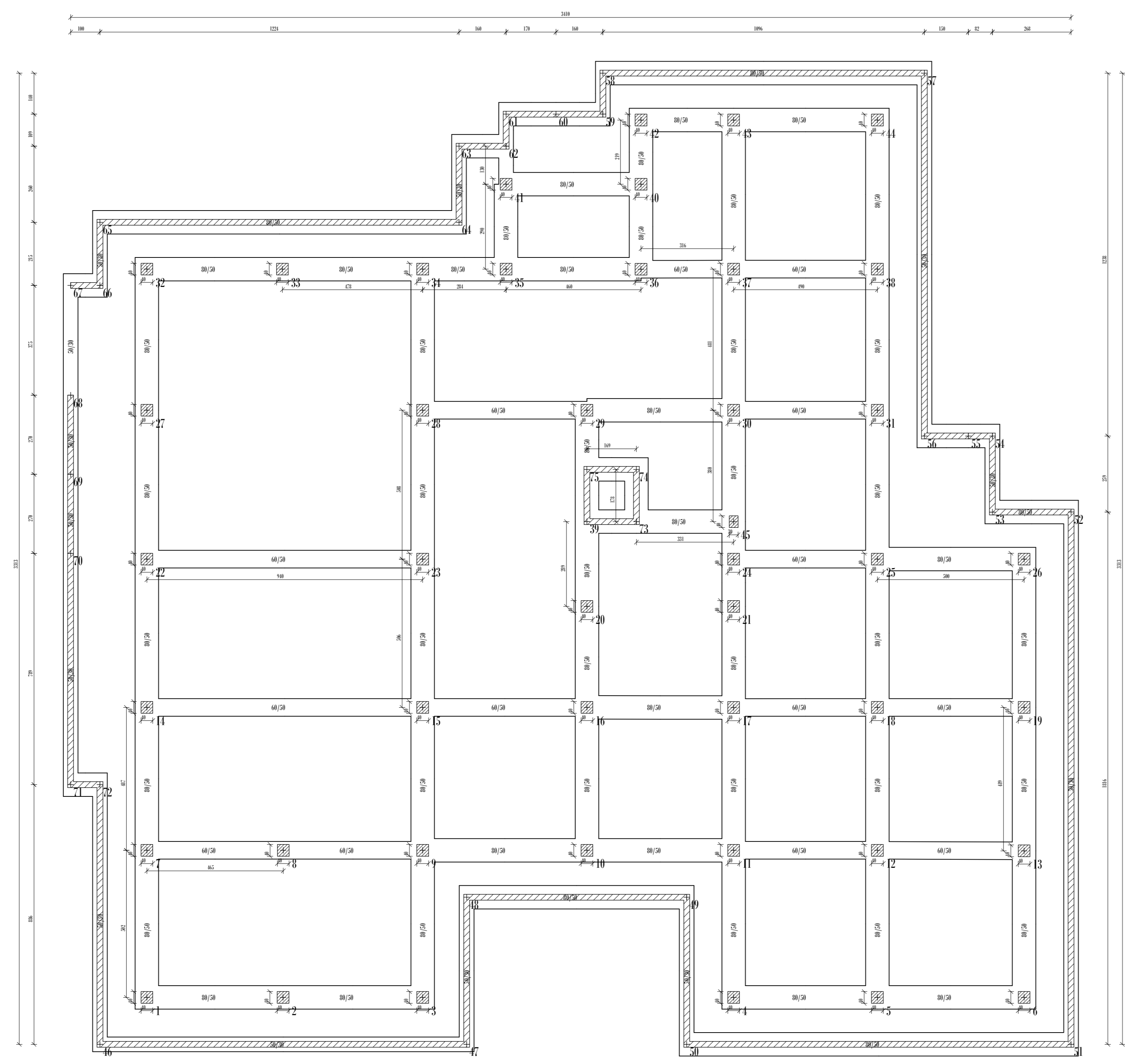
PIANTA IMPALCATO QUOTA mc 0.00
