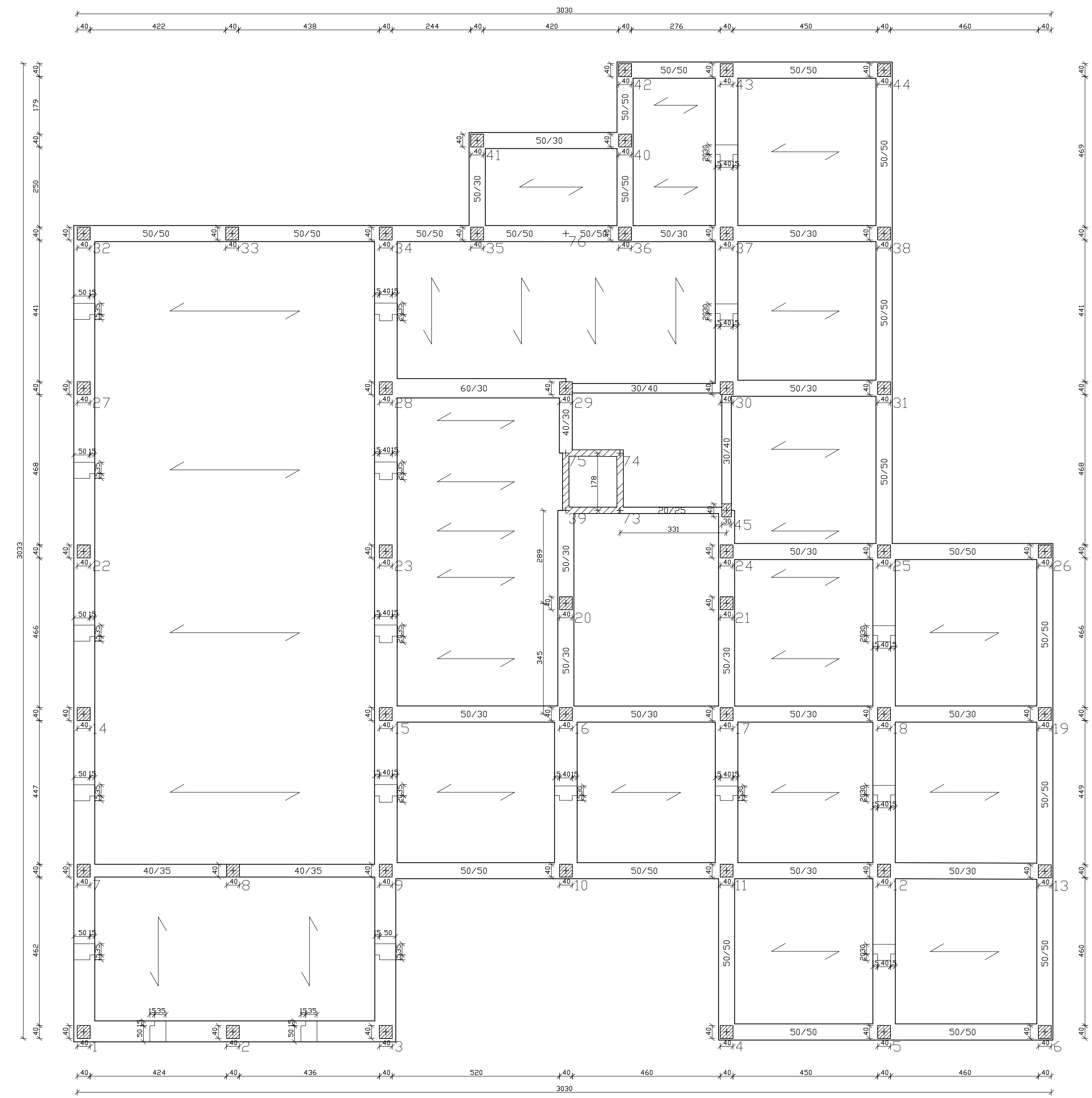
PIANTA IMPALCATO QUOTA m: 3.80
