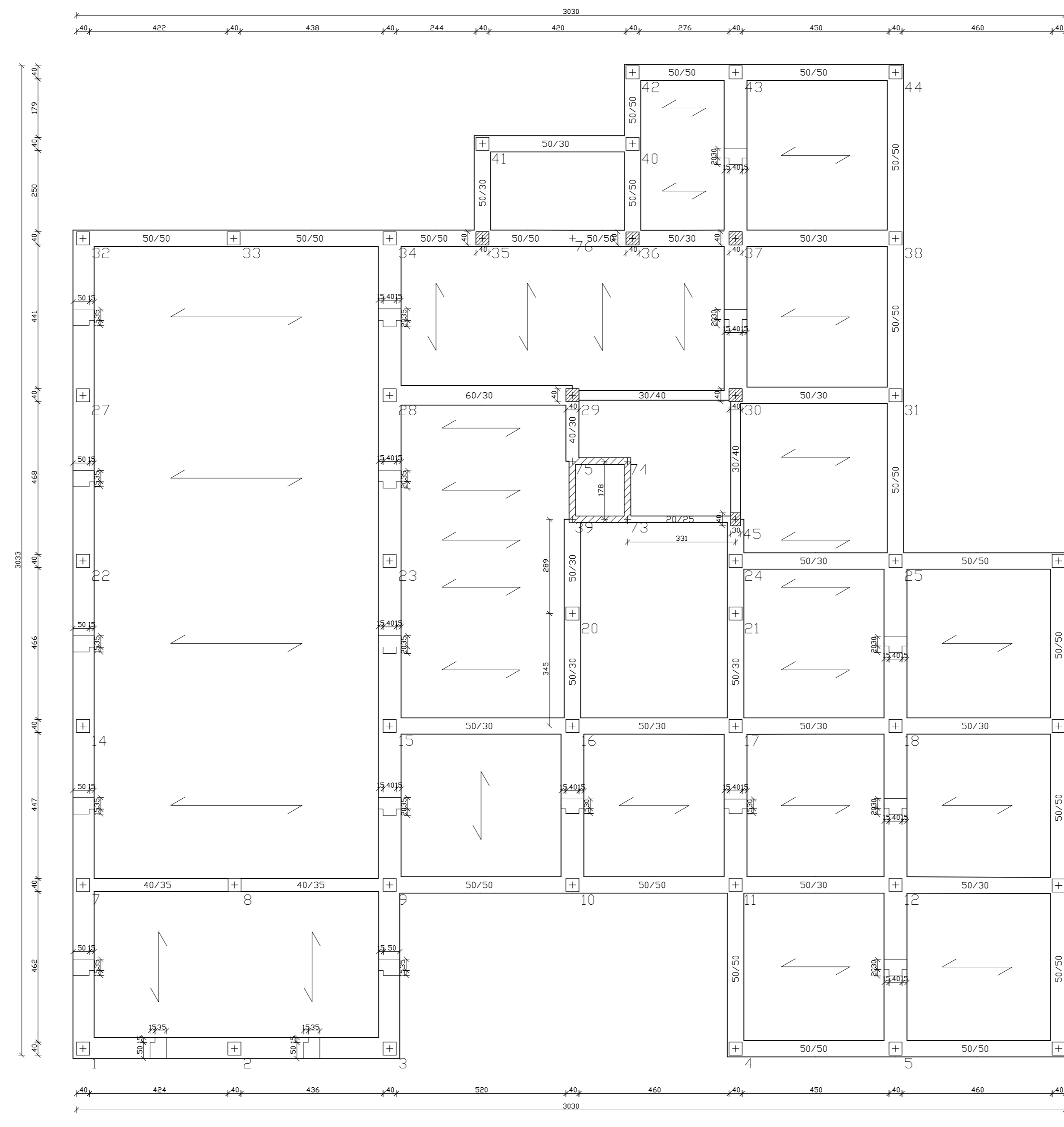
PIANTA IMPALCATO QUOTA m: 7.30
